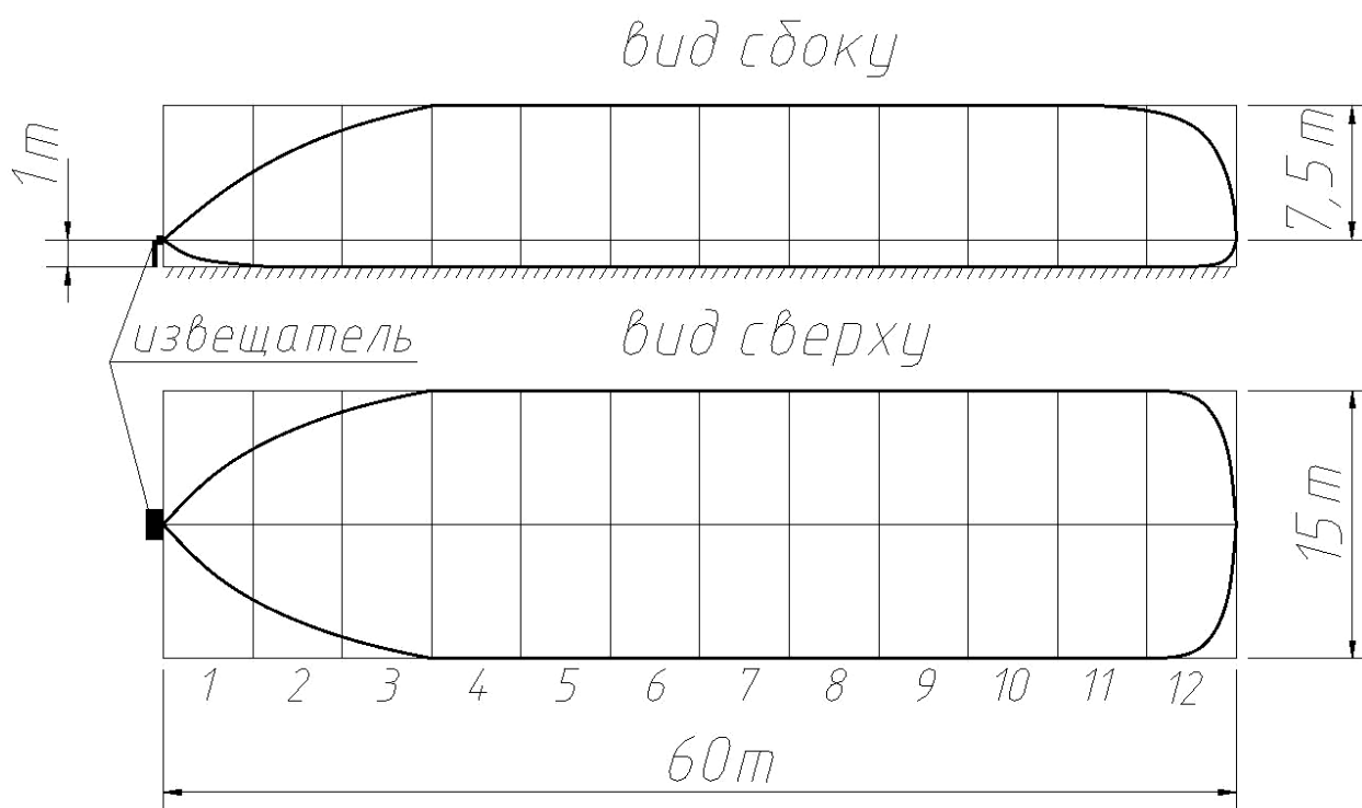
Рисунок 12.1 Форма и размеры зоны обнаружения извещателя для варианта исполнения «объем» при установке на высоте 1 метр.
