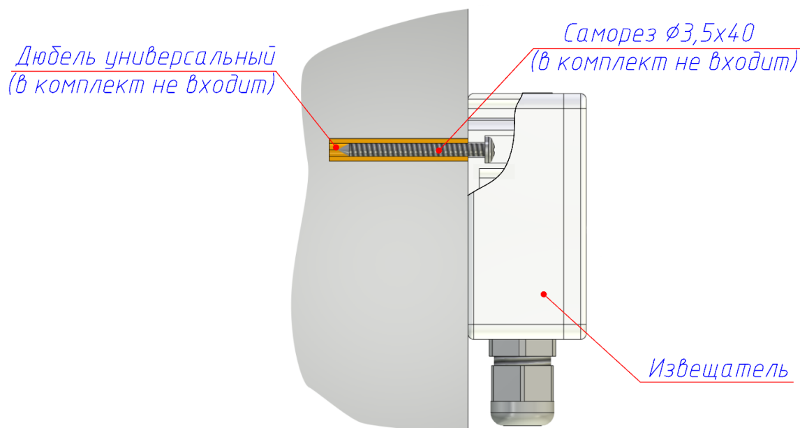
Рисунок 2.5 – Крепление извещателя
