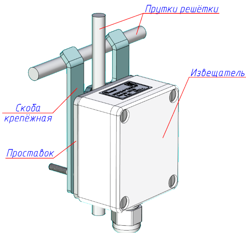
Рисунок 2.1 – Крепление извещателя на решетке из прутка
