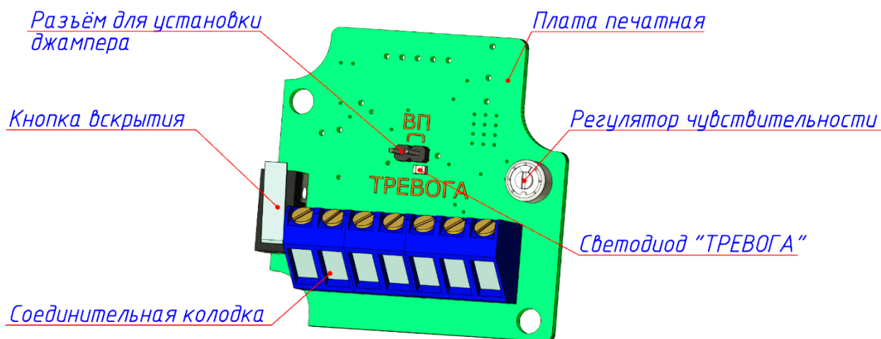
Рисунок 1.2 – Конструкция платы
