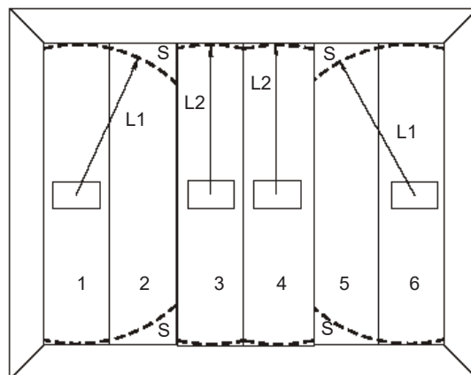
Рисунок 7 – Защита немонолитной конструкции
