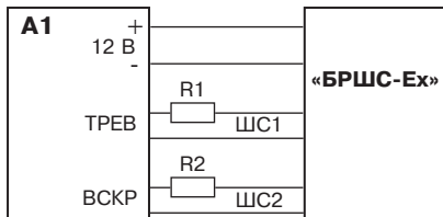
Рисунок 2 — Схема подключения извещателя с раздельной передачей извещений «Тревога» и «Вскрытие»
