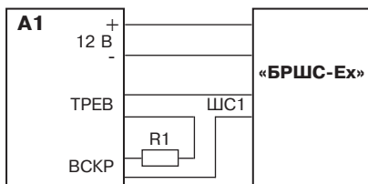
Рисунок 1 — Схема подключения извещателя с объединенной передачей извещений «Тревога» и «Вскрытие»
