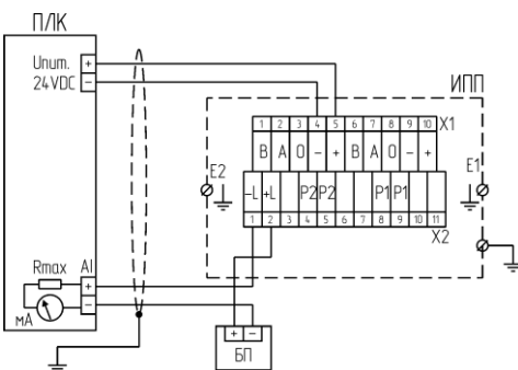
б) извещатель в качестве источника тока
