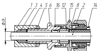
и) монтаж бронированным кабелем в металлорукаве в кабельном вводе KBMB
