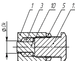
е) монтаж заглушки 3Г
