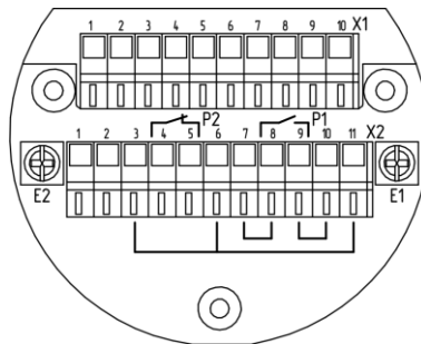
Рисунок Б.2 - Плата клемм извещателя IPII-07ea-RS-HART.
