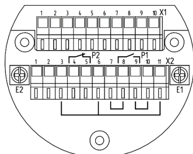
б) Плата клемм извещателя ИПП-07еа-RS-4/20мА
