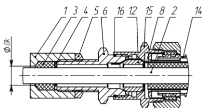
и) монтаж бронированным кабелем в металлорукаве в кабельном вводе KBМВ
