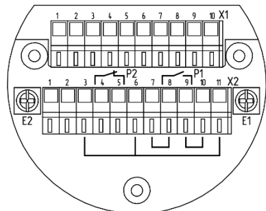
б) Плата клемм извещателя ИПП-07ea-RS-4/20мА
