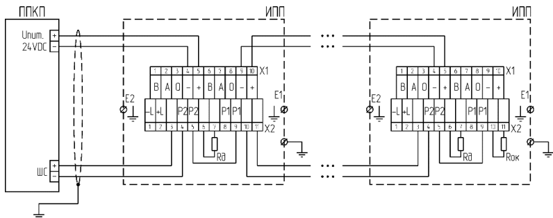
б) схема подключения извещателя ИПП-07ea-RS-4/20мА
