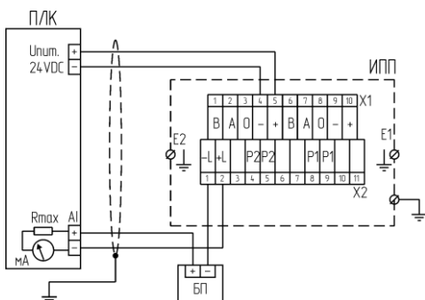
а) извещатель в качестве потребителя тока
