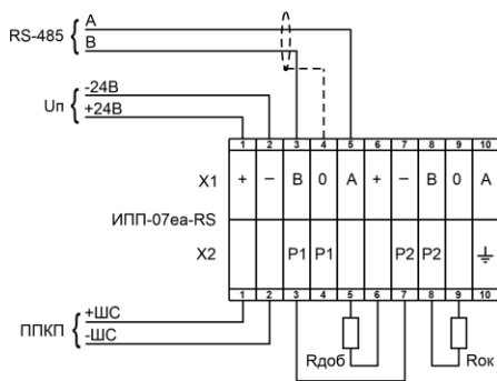
а) схема подключения извещателя ИПП-07еа-RS
