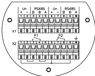
а) Плата клемм извещателя ИПП-07еа-RS
