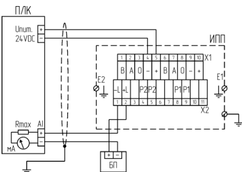
б) извещатель в качестве источника тока
