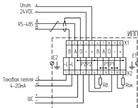
б) схема подключения извещателя ИПП-07еа-RS-4/20мА
