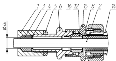
и) монтаж бронированным кабелем в металлорукаве в кабельном вводе КВВМ
