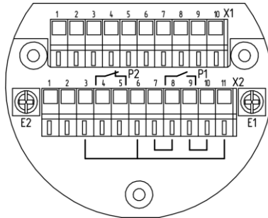
Рисунок Б.2 - Плата клемм извещателя ИПП-07еа-RS-HART.
