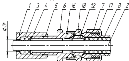
з) монтаж бронированным кабелем в кабельном вводе КВВУ
