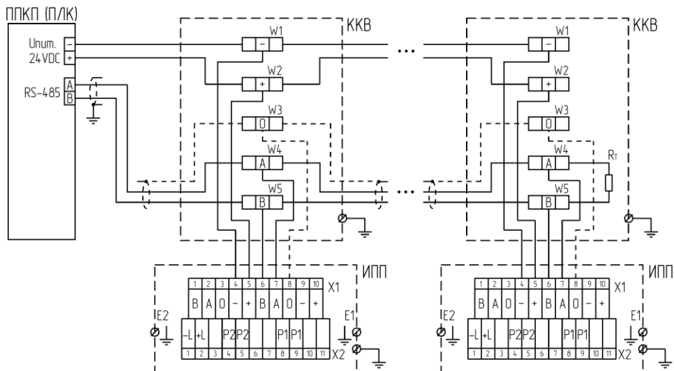
Рисунок Б.13 - Вариант подключения извещателей к интерфейсу RS-485 через клеммные коробки типа KKB-07е.
