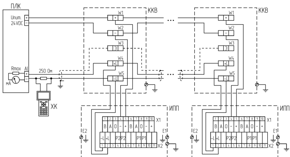
Рисунок Б.14 - Вариант подключения извещателей к интерфейсу HART через клеммные коробки типа KKB-07е.
