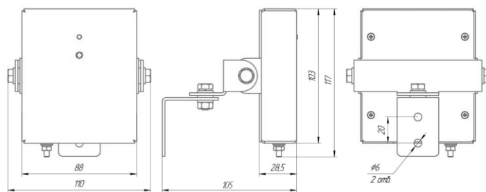
«C2000-Спектрон-207-Exi-M», «C2000-Спектрон-207-Exm-M»
