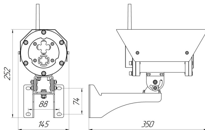
Рисунок 2.4 Монтажные размеры «C2000P-Спектрон-609-Exd-M» и «C2000P-Спектрон-609-Exd-H»
