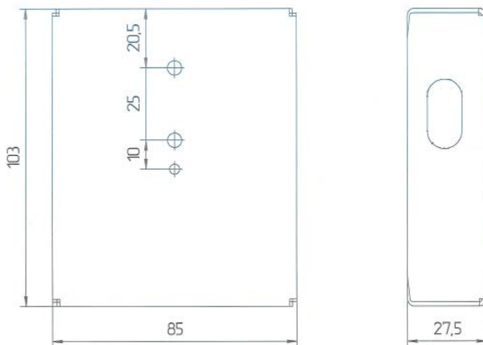
Рисунок А2 – Габаритные и установочные размеры Спектрон-202-Exm/Exi-M, -202-Exm/Exi-H
