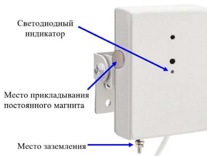
Рисунок 2. Внешний вид извещателей: Спектрон-204 в металлическом корпусе
