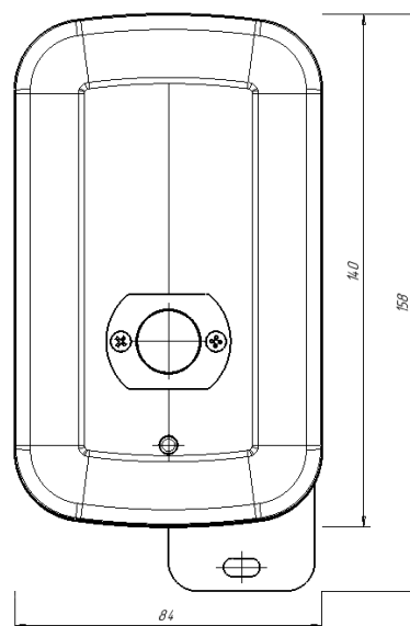
Рисунок А1 – Габаритные и установочные размеры Спектрон-204
