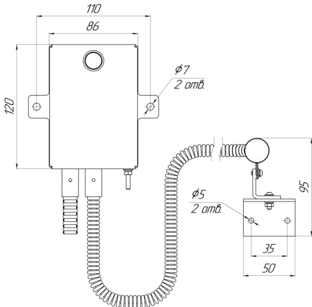
Рис. 1 – Извещатель
