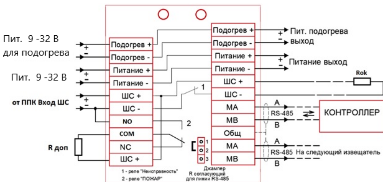
Рисунок 8 – Схема подключения
