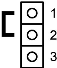
Рисунок 9 – Установка джампера согласующего резистора
