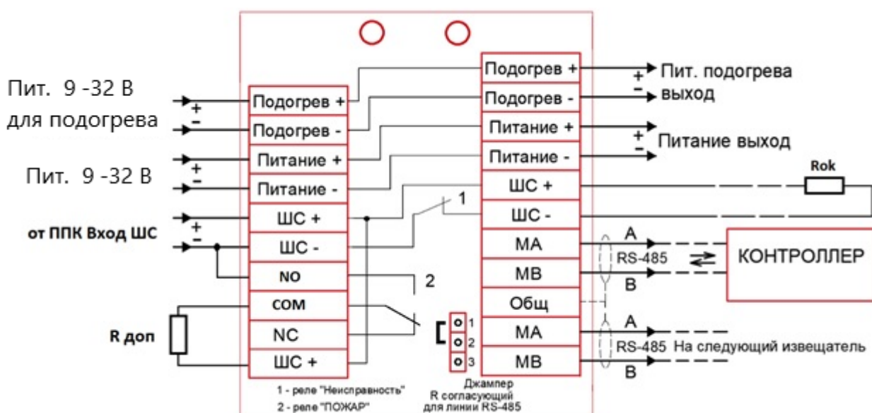
Рисунок 8 – Схема подключения
