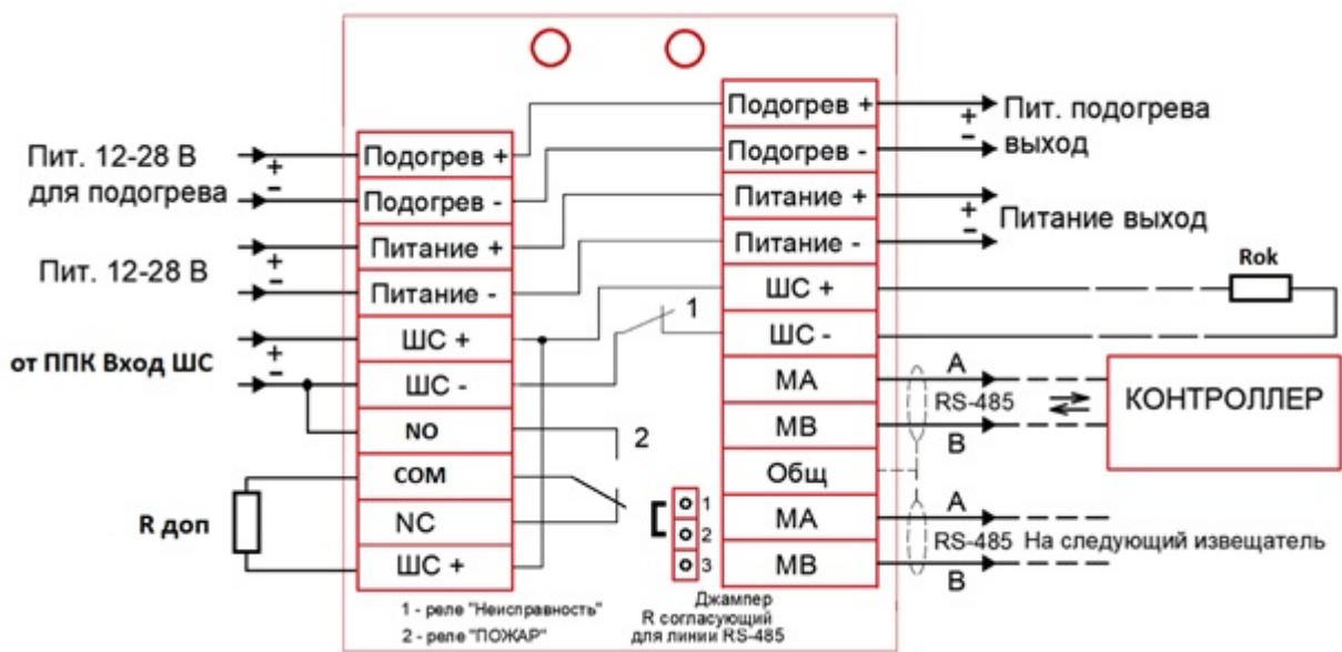
Рисунок 7 – Схема подключения
