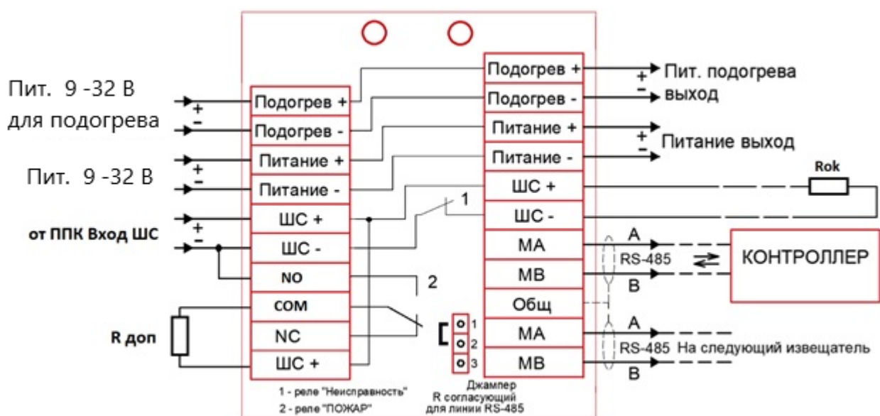
Рисунок 8 – Схема подключения
