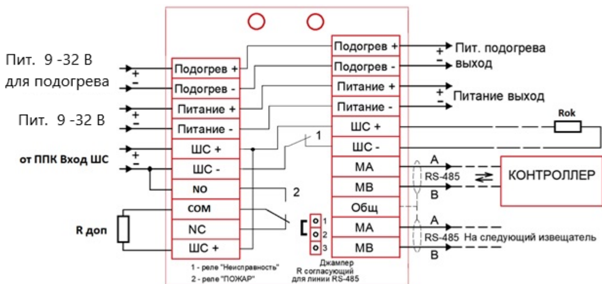
Рисунок 8 – Схема подключения
