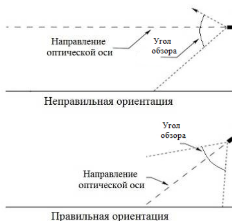
Рисунок 4 – Установка извещателя по отношению к горизонту
