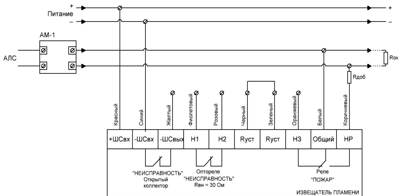
Рисунок Б8 – 4-х проводная схема подключения к АМ-1 без использования режима «НЕИСПРАВНОСТЬ»
