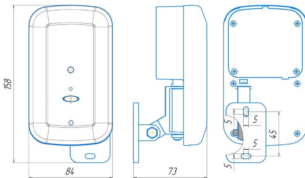
Рисунок А1 – Габаритные размеры Спектрон-601-С
