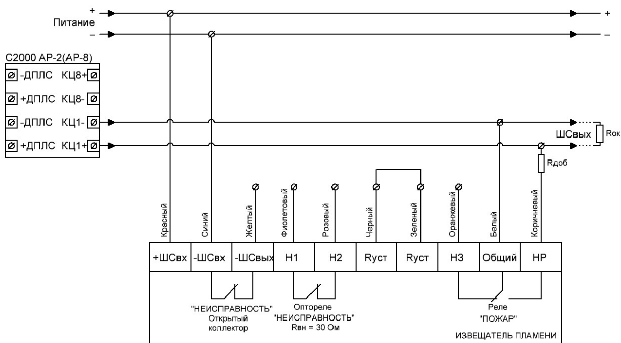
Рисунок Б6 – 4-х проводная схема подключения к С2000-АР2 (АР-8) без использования режима «НЕИСПРАВНОСТЬ»
