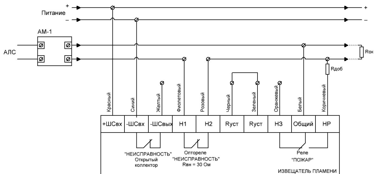
Рисунок Б7 – 4-х проводная схема подключения к АМ-1 с использованием режима «НЕИСПРАВНОСТЬ»
