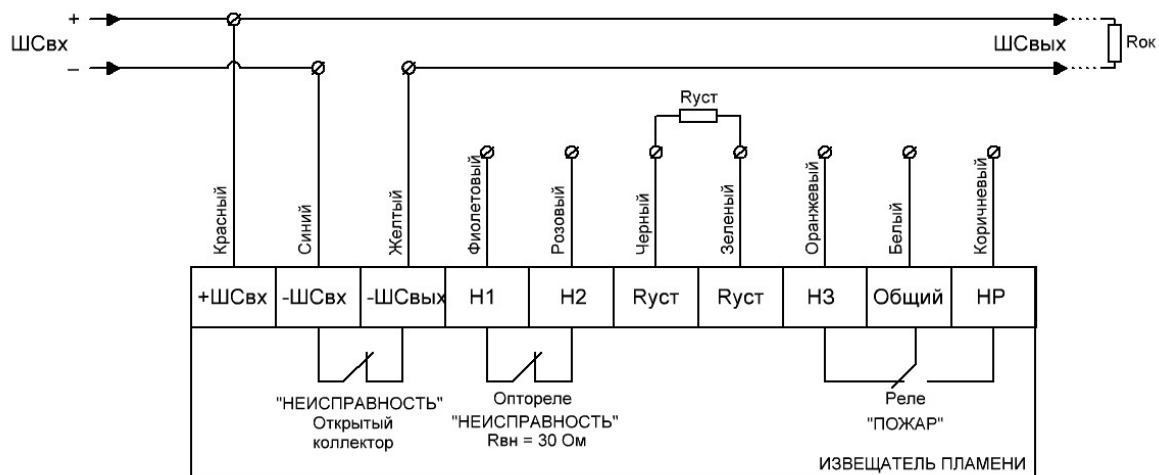
Рисунок Б1 – 2-х проводная схема подключения с использованием режима «НЕИСПРАВНОСТЬ»
