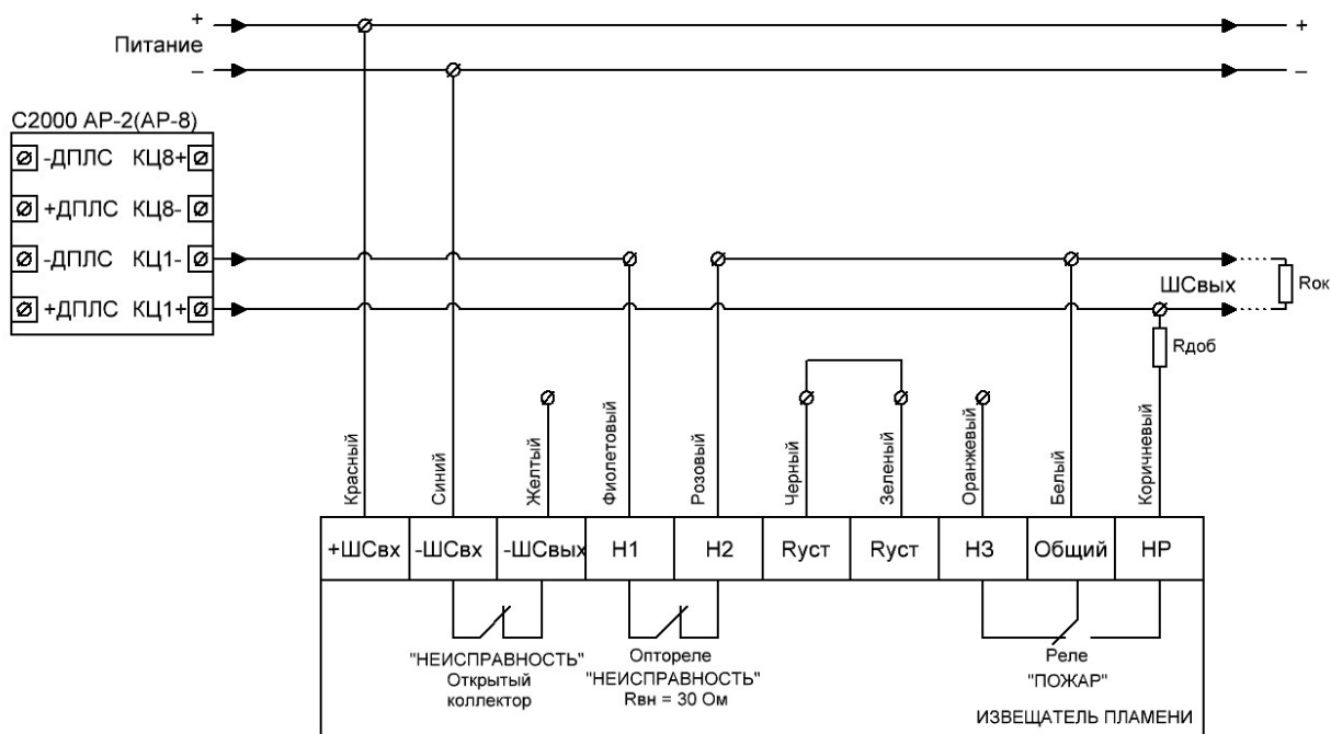
Рисунок Б5 – 4-х проводная схема подключения к С2000-АР2 (АР-8) с использованием режима «НЕИСПРАВНОСТЬ»
