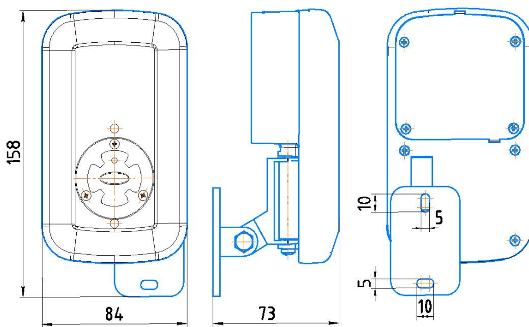
Рисунок А2 – Габаритные размеры Спектрон-601-Exi-C, -601-Exm-C
