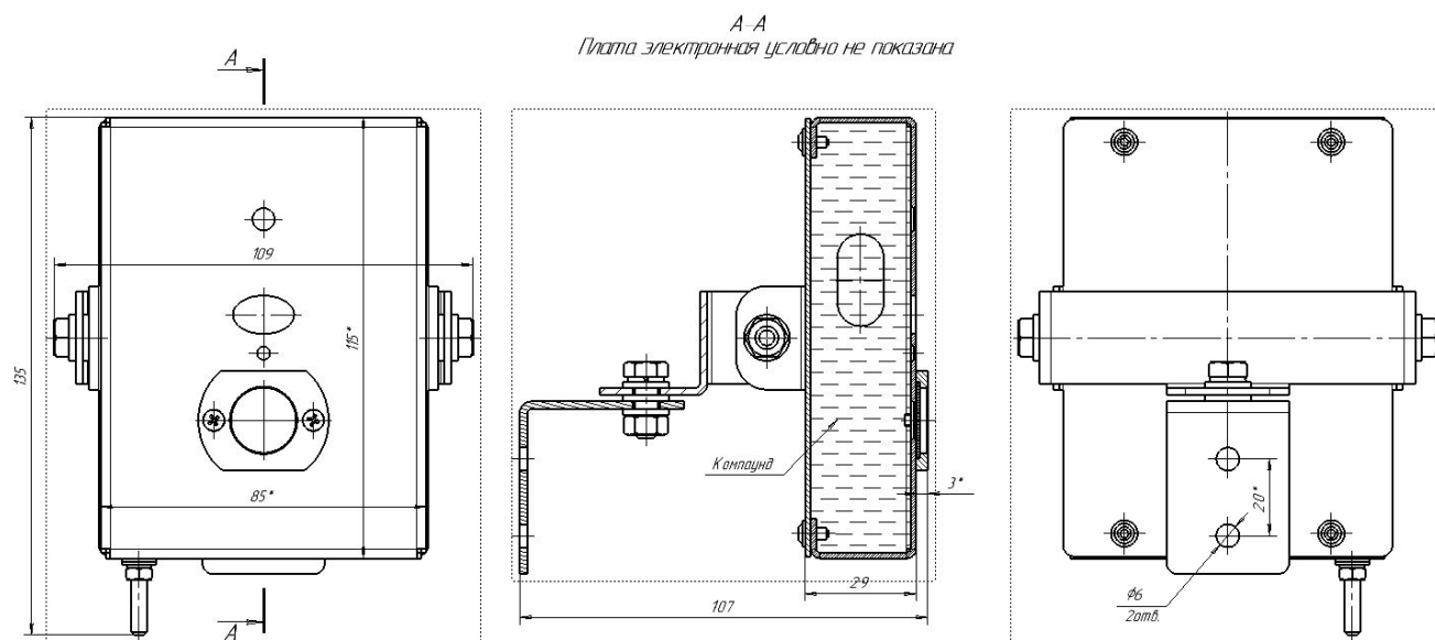
Рисунок А1 – Габаритные размеры Спектрон-601-М
