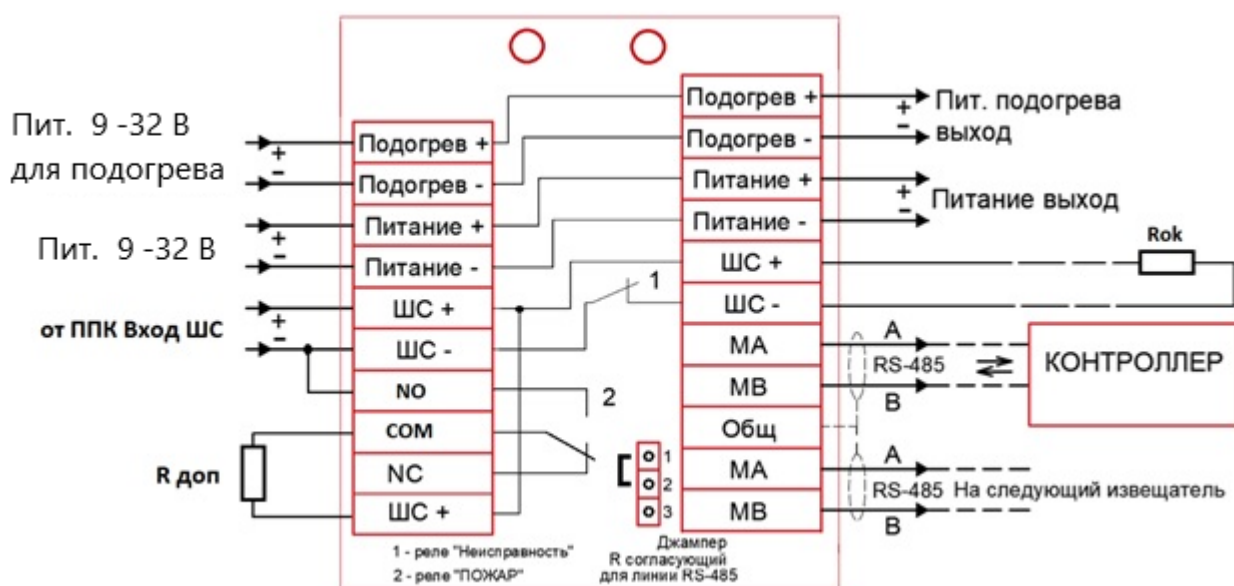
Рисунок 5 – Схема подключения
