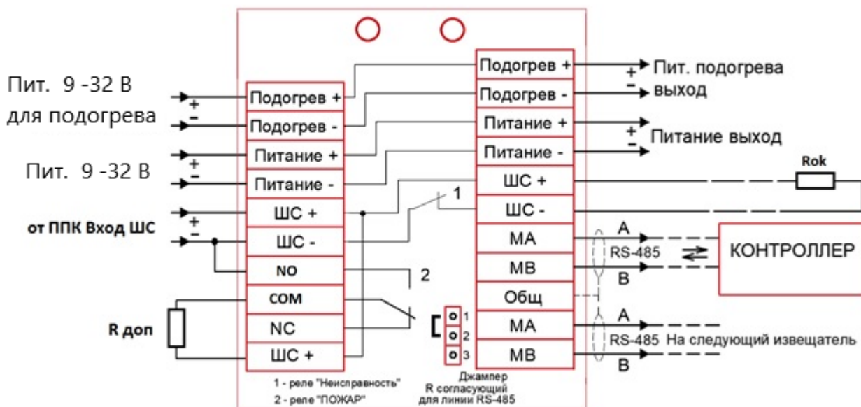
Рисунок 5 – Схема подключения
