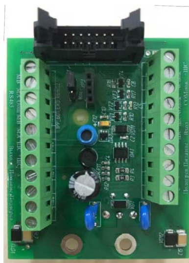
Рисунок 9 – Клеммная плата извещателя
