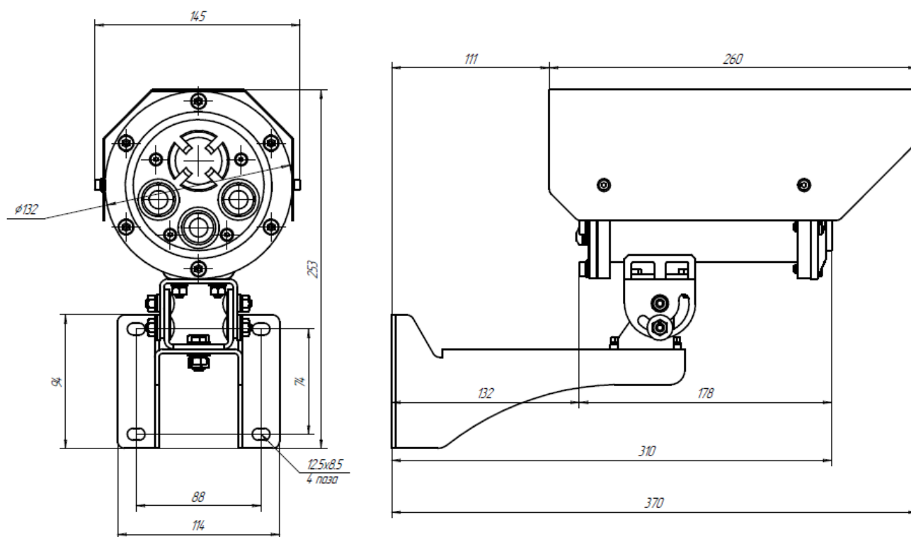
Рисунок А2. Габаритные размеры Спектрон-801-Exd-M/H-HART
