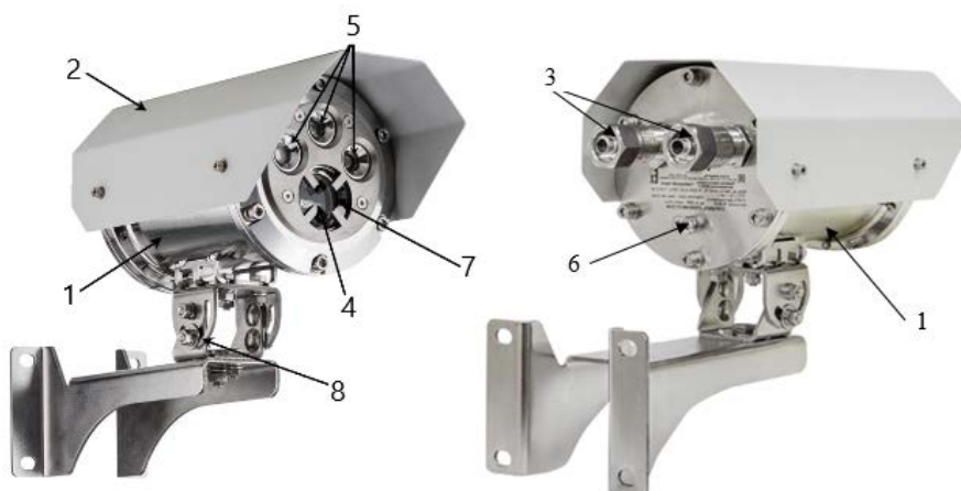
1 – корпус извещателя; 2 – солнцезащитный козырек; 3 – кабельные вводы; 4 – светодиодные индикаторы; 5 – приемники ИК-излучения; 6 – место заземления; 7 – место поднесения магнита; 8 – крепежно-юстировочное устройство
