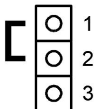
Рисунок Б2 – Установка джампера согласующего резистора Переключатель в положении «1-2» – согласующий резистор подключен . Переключатель в положении «2-3» – согласующий резистор отключен .
