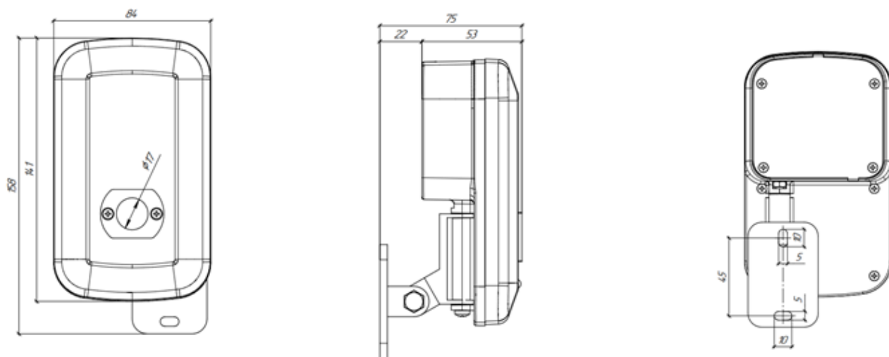
Рисунок А1 – Габаритные размеры Спектрон-Ехі, -801-Ехм.
