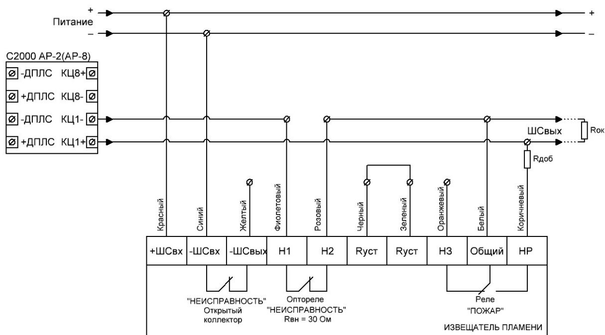
Рисунок Б5 – 4-х проводная схема подключения к C2000-AP2 (AP-8) с использованием режима «НЕИСПРАВНОСТЬ»
