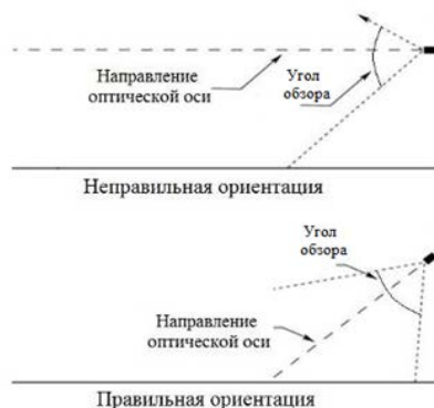
Рисунок 3 – Установка извещателя по отношению к горизонту
