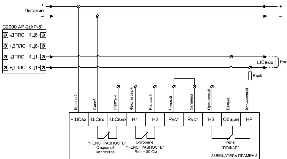
Рисунок Б6 – 4-х проводная схема подключения к C2000-AP2 (AP-8) без использования режима «НЕИСПРАВНОСТЬ»
