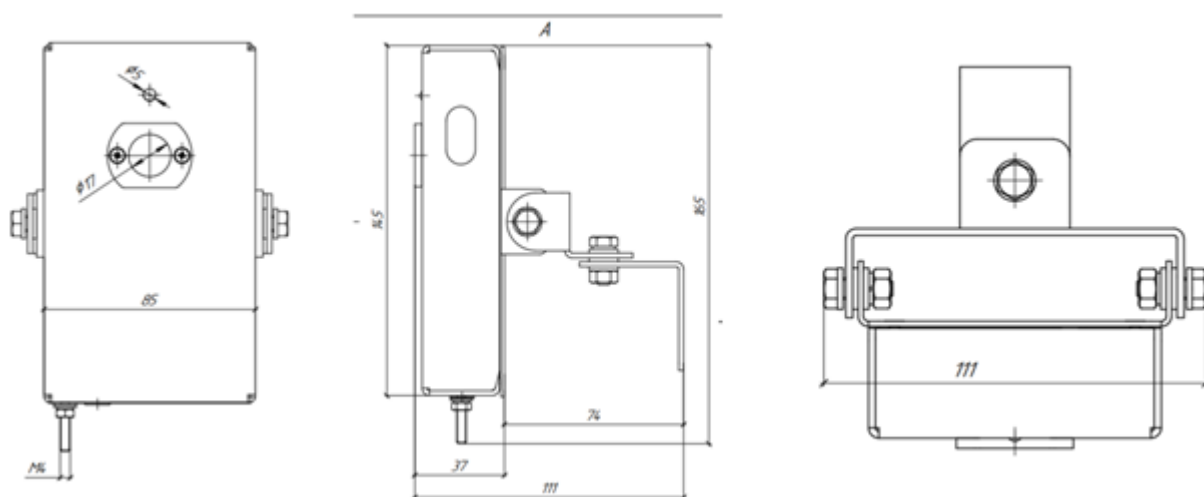
Рисунок А2 – Габаритные размеры Спектрон-801-Ехi-М, -801-Ехi-Н, -801-Ехm-М, -801-Ехm-Н
