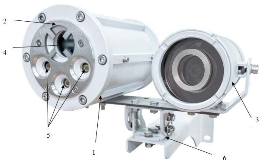
1 – корпус извещателя; 2 – место поднесения магнита; 3 – корпус видеомодуля; 4 – светодиодный индикатор; 5 – приемник ИК-излучения; 6 – крепежно-юстировочный кронштейн.
