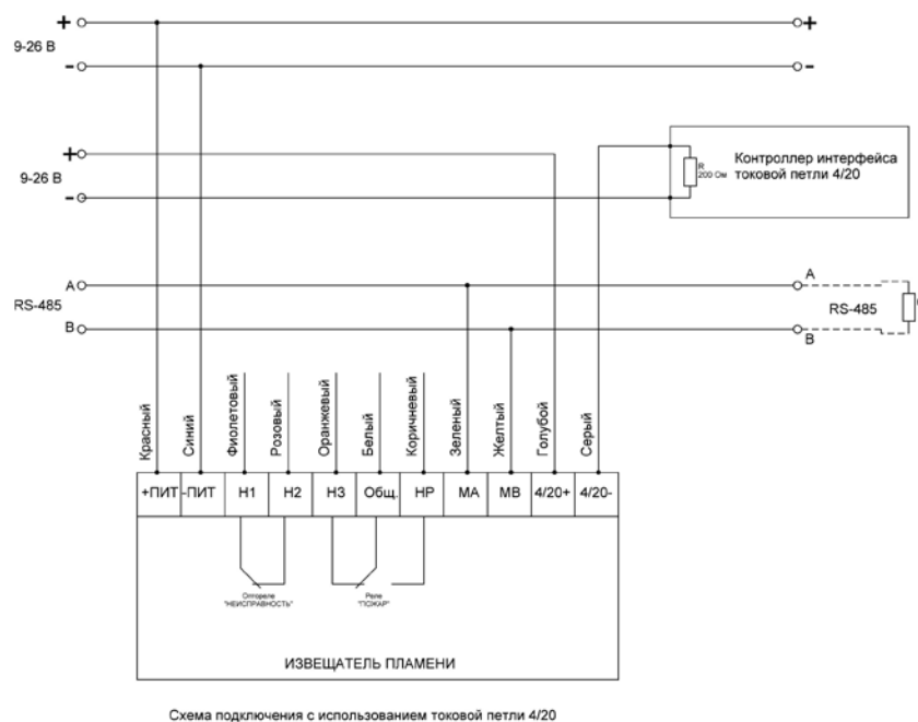
Рисунок Б3 – схема подключения с использованием токовой петли 4/20
