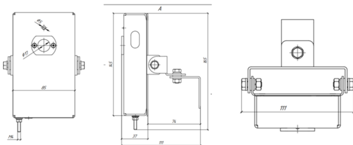
Рисунок А2 – Габаритные размеры Спектрон-804-Ехі-М, -804-Ехі-Н, -804-Ехм-М, -804-Ехм-Н
