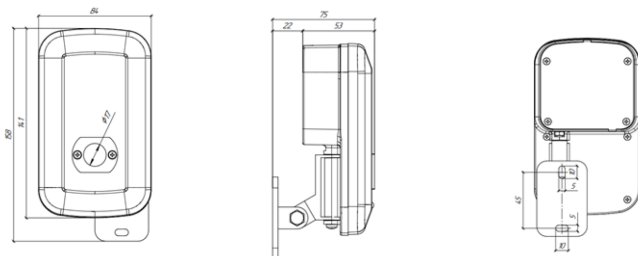
Рисунок А1 – Габаритные размеры Спектрон-Ехі, -804-Ехм.
