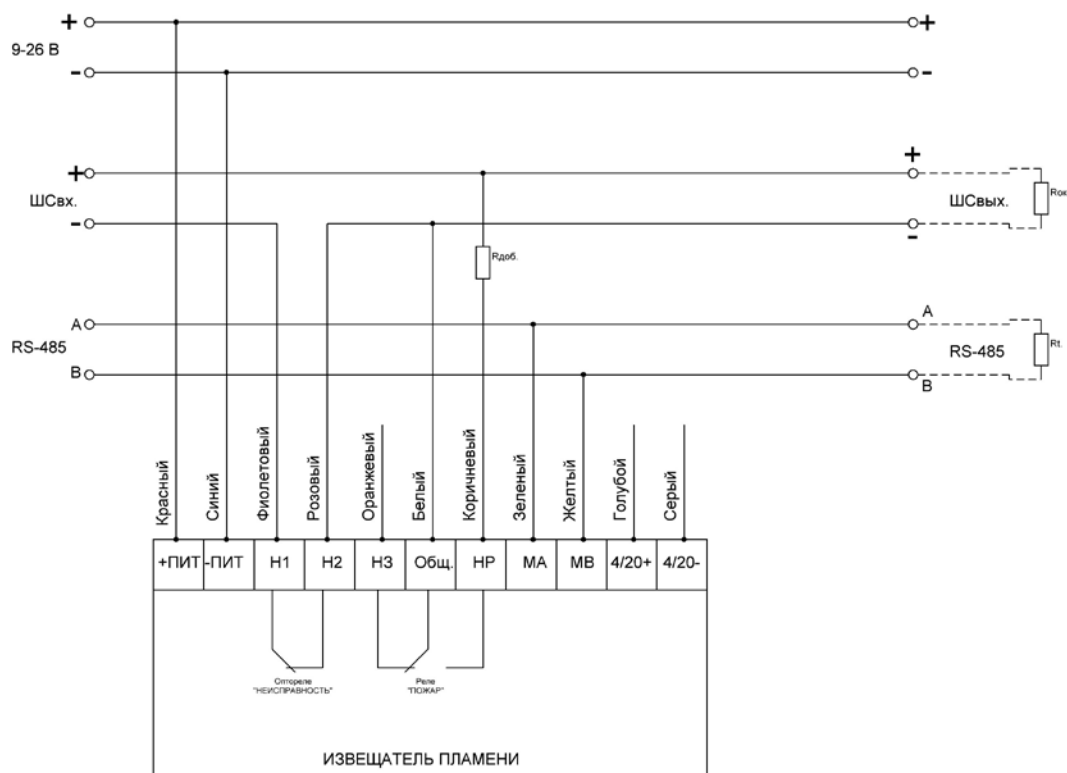
Рисунок Б1 – 4-х проводная схема подключения с использованием режима «НЕИСПРАВНОСТЬ»
