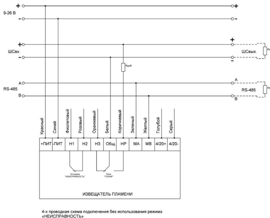
Рисунок Б2 – 4-х проводная схема подключения без использования режима «НЕИСПРАВНОСТЬ»
