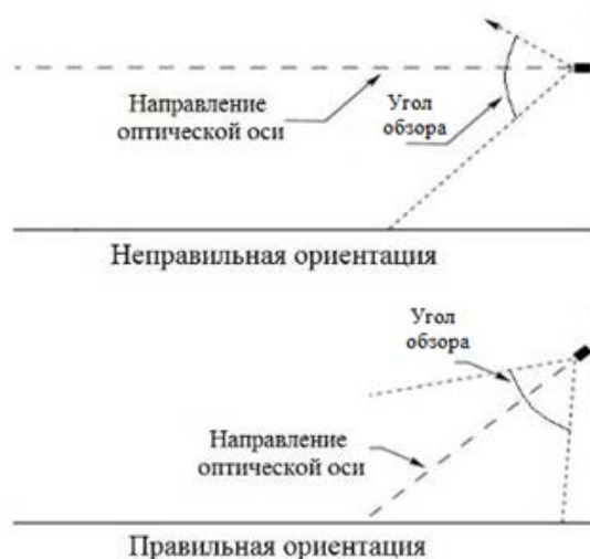
Рисунок 3 – Установка извещателя по отношению к горизонту
