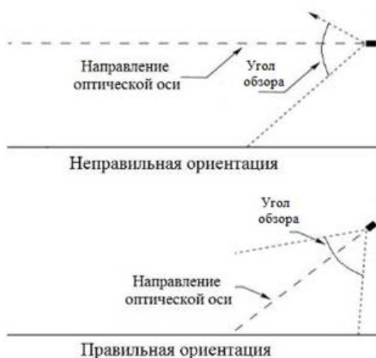
Рисунок 3 – Установка извещателя по отношению к горизонту
