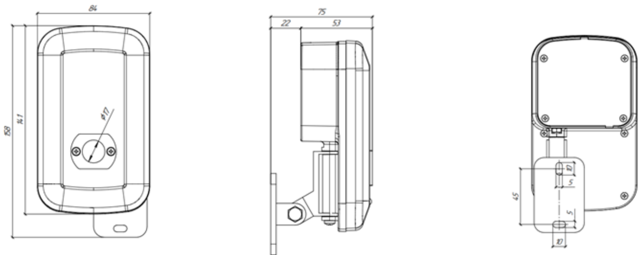
Рисунок А1 – Габаритные размеры Спектрон-Ехi, -804-Exm.
