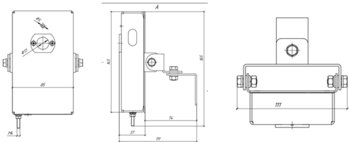
Рисунок А2 – Габаритные размеры Спектрон-804-Exi-M, -804-Exi-H, -804-Exm-M, -804-Exm-H
