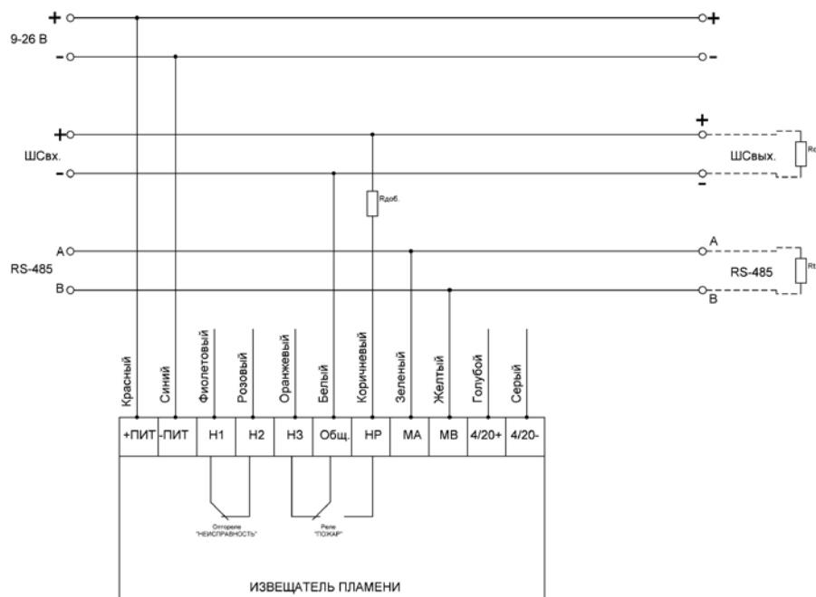
4-х проводная схема подключения без использования режима «НЕИСПРАВНОСТЬ»
