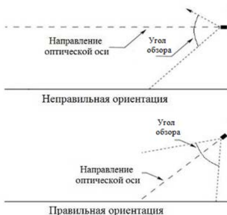
Рисунок 3 – Установка извещателя по отношению к горизонту
