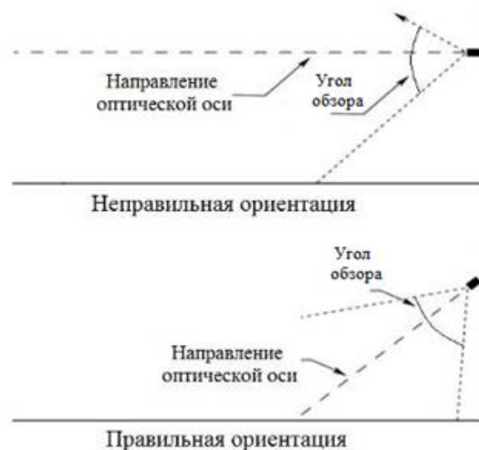
Рисунок 3 – Установка извещателя по отношению к горизонту
