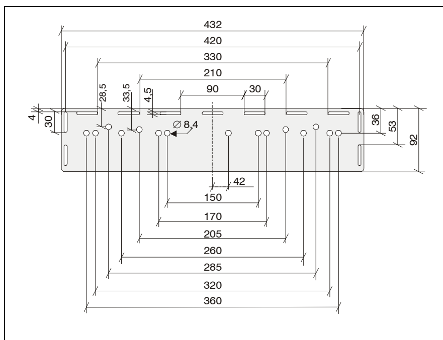
Рис. 5.9: Положение отверстий на крепежной пластине Тип MT-1
