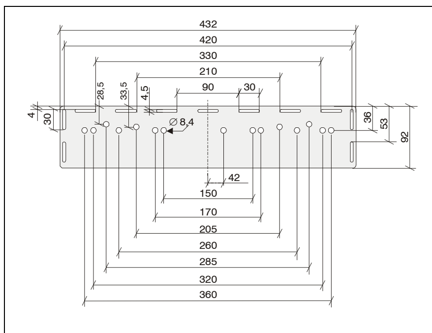
Рис. 5.9: Положение отверстий на крепежной пластине Тип МТ-1
