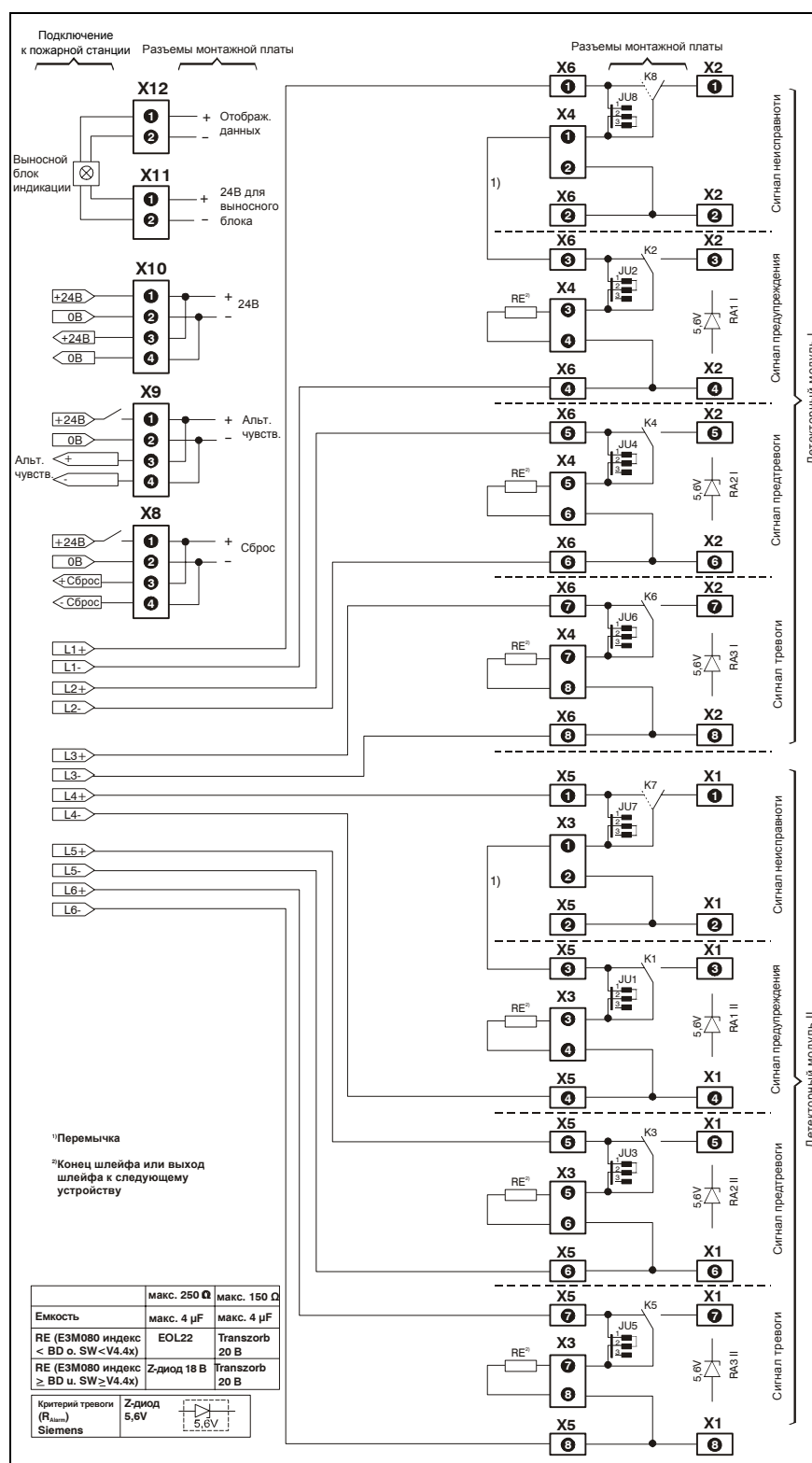
Рис. 5.13: Подключение TITANUS® через безпотенциальные контакты с кнопкой сброса
