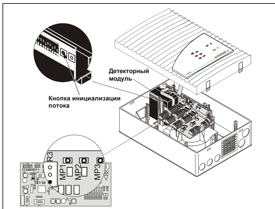
Рис. 7.2: Настройка датчика воздушного потока без учёта давления воздуха в TITANUS®
