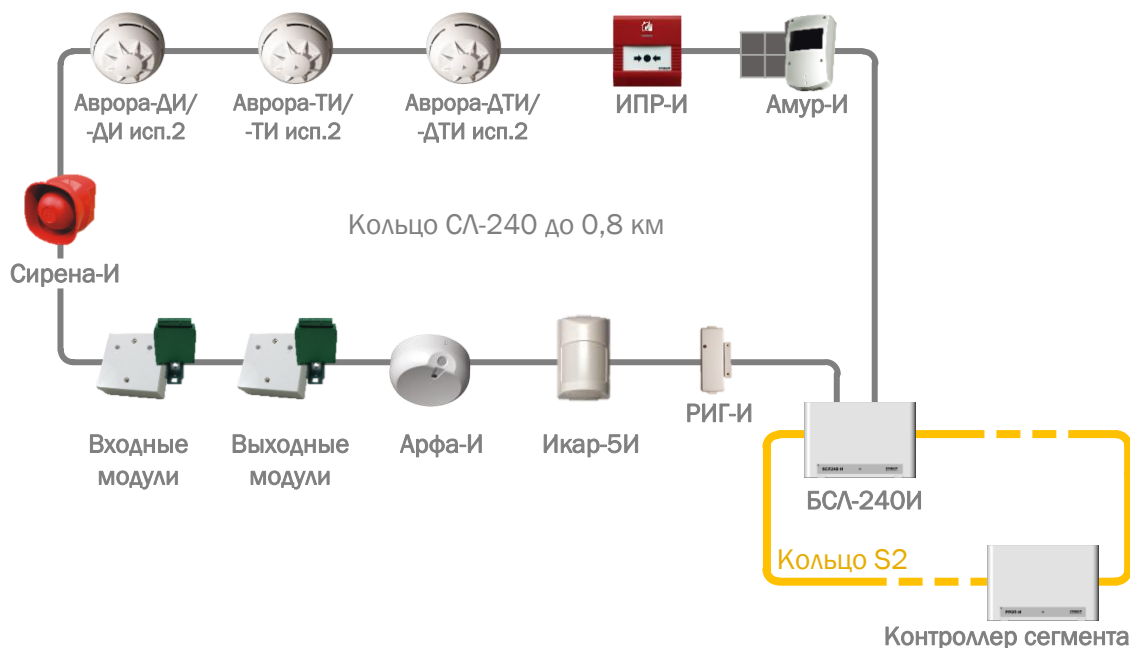
Рисунок 17 Оборудование СЛ-240
