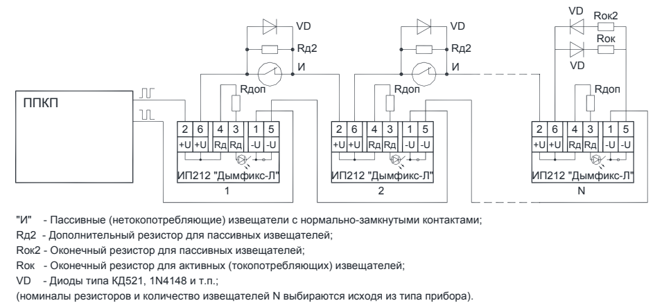
Рис.В.2. Схема подключения извещателей ИП212 «ДЫМФИКС -Л» в шлейф сигнализации со знакопеременным импульсным напряжением
