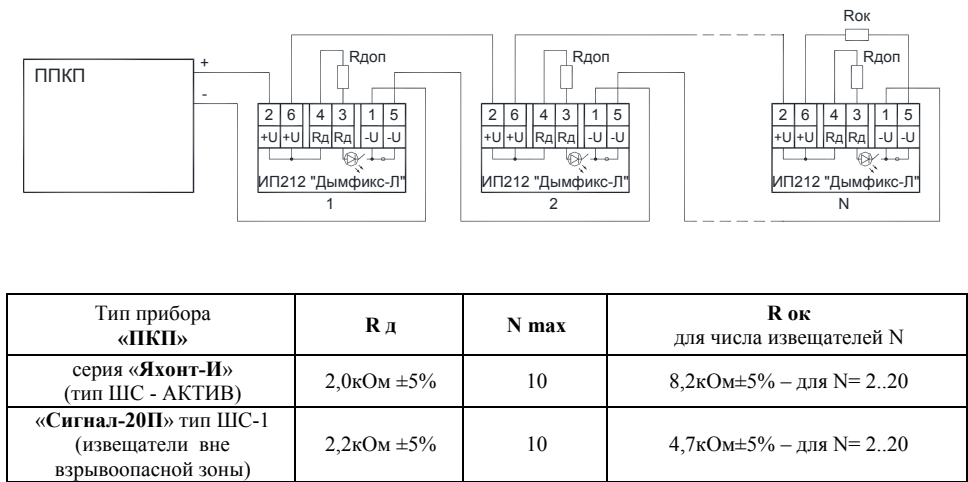
Рис.В.1. Схема подключения извещателей ИП212 «ДЫМФИКС - Л» в однополярный шлейф сигнализации с контролем исправности извещателей
