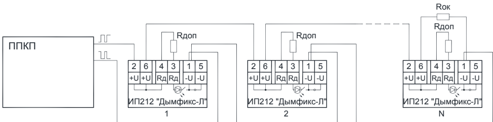
Рис.В.3. Схема подключения извещателей ИП212 «ДЫМФИКС -Л» без передачи прибору сигнала о неисправности извещателей (только визуальный сигнал). Номиналы Рд и Рок – см. рис.В.1.
