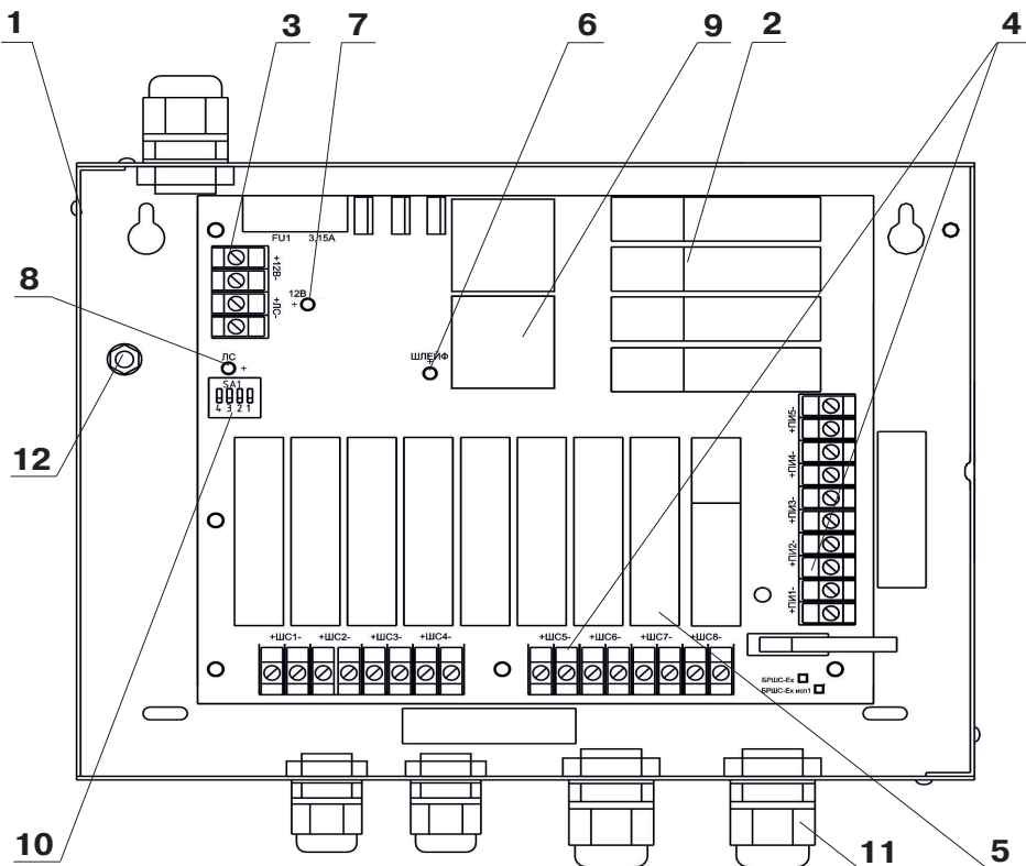
Рисунок 10 – «БРШС-Ех» исполнение 1, вид со снятой крышкой
